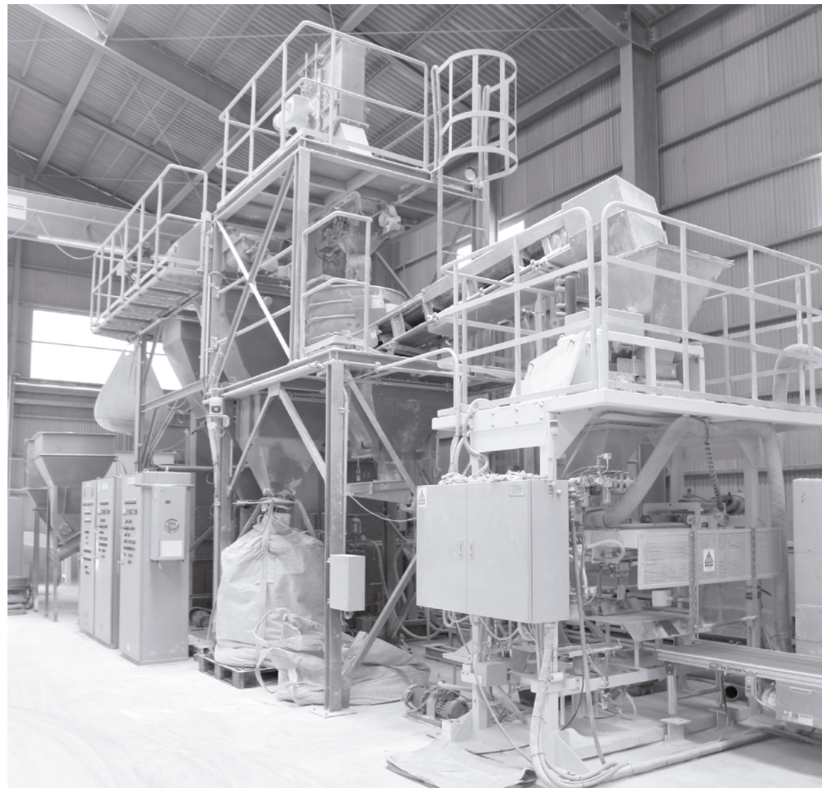
工場内でもひととき大きく鎮座しているこの機械は粉の石灰を粒状に固めるもの。この機械だけで1億円以上もするとのこと。
